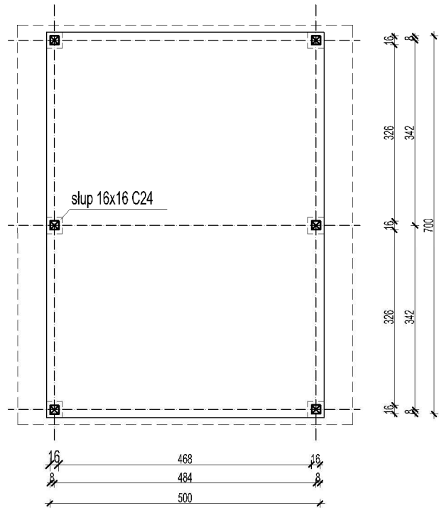
RZUT PRZYZIEMIA 1:100
